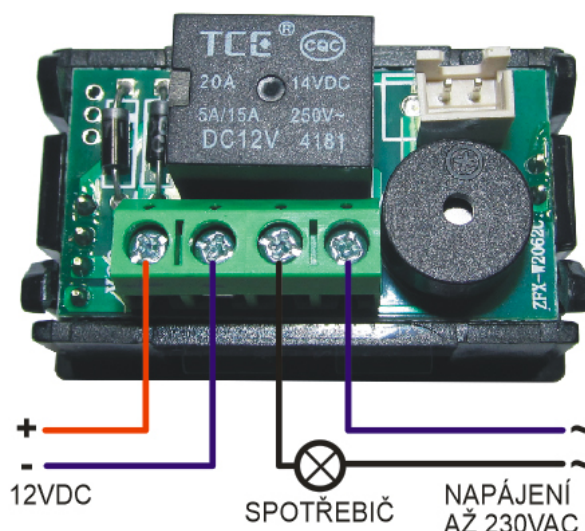
Zapojení pro spotřebič s rozdílným napájením.
