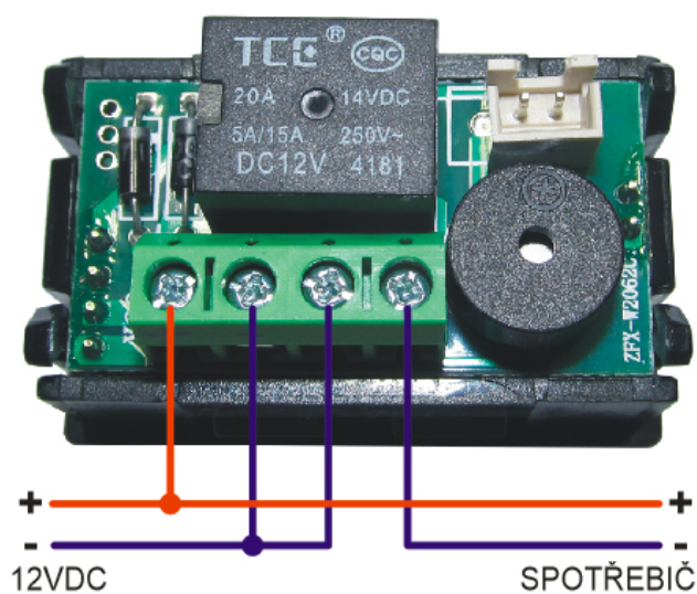
Zapojení pro spotřebič s napájením 12VDC.
